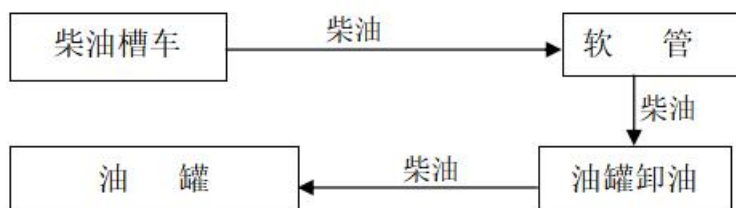
图 2.2-2 柴油卸油工艺流程图
