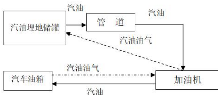
图 2.2-3 汽油加油工艺流程图
