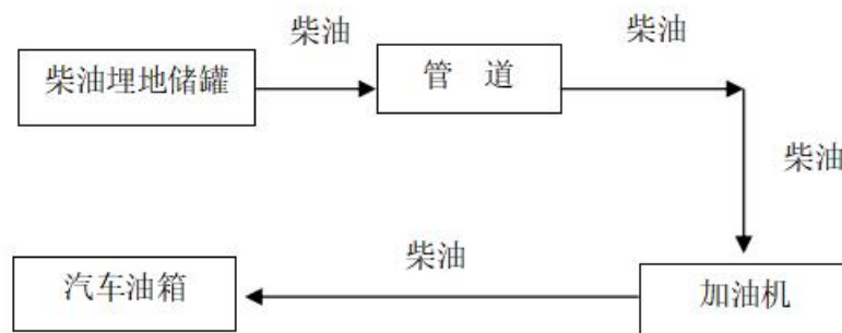
图 2.2-4 柴油加油工艺流程图
