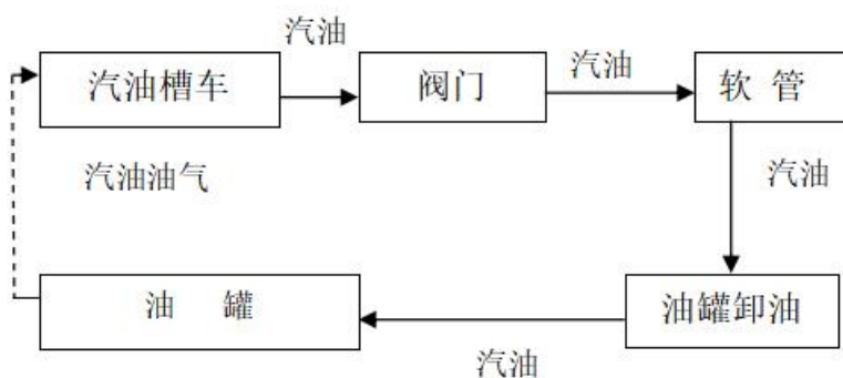
图 2.2-1 汽油卸油工艺流程图
