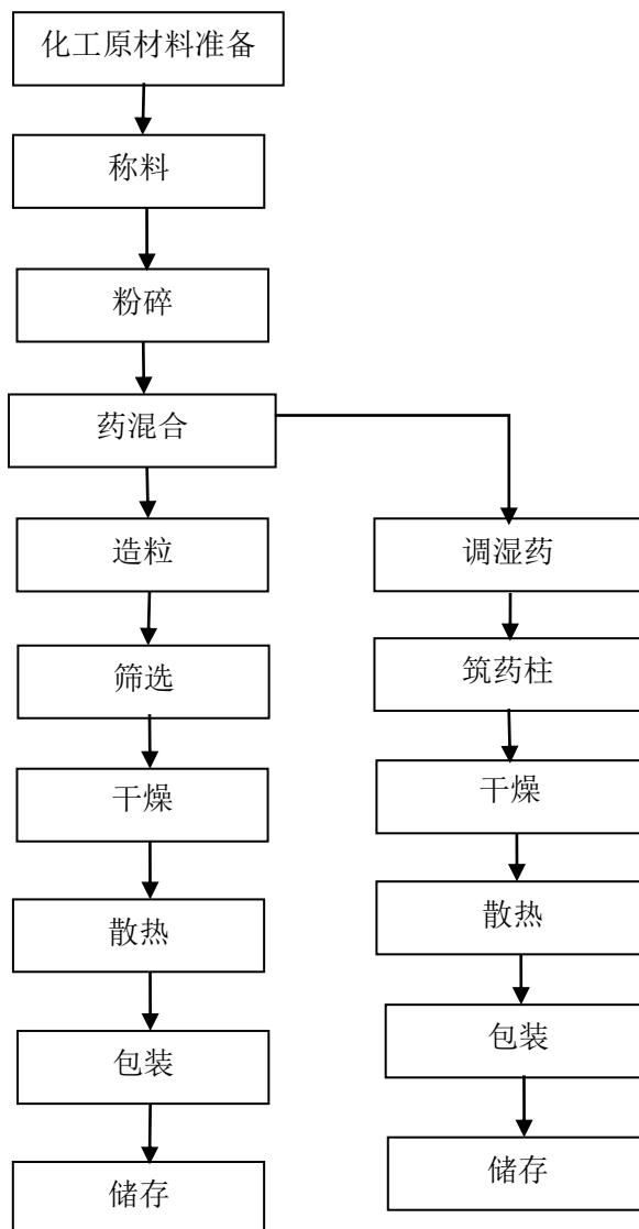
图 2.4-1 亮珠药柱生产工艺流程图
