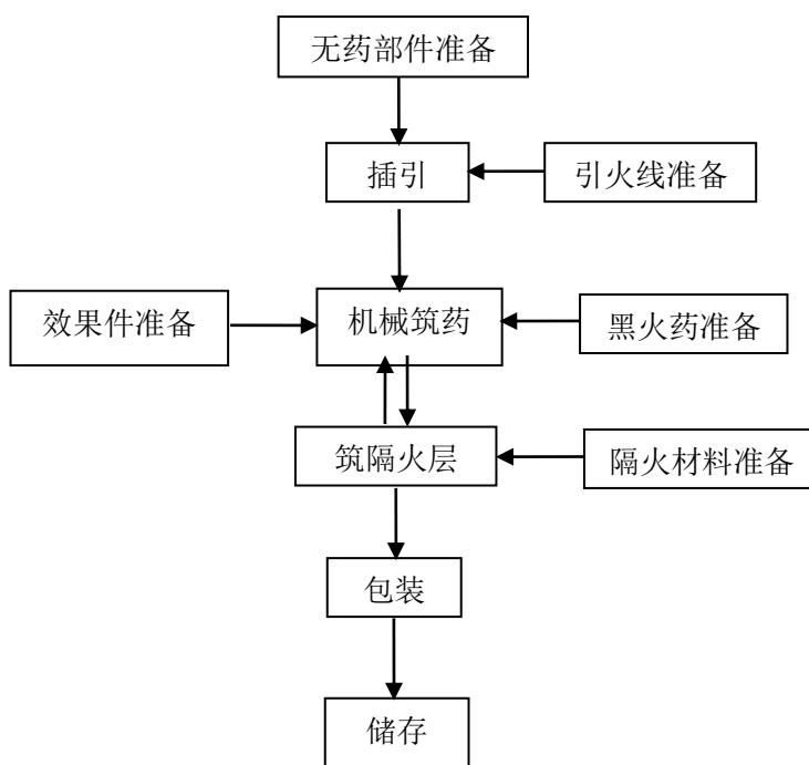
图 2.4-4 喷花类产品生产流程图
