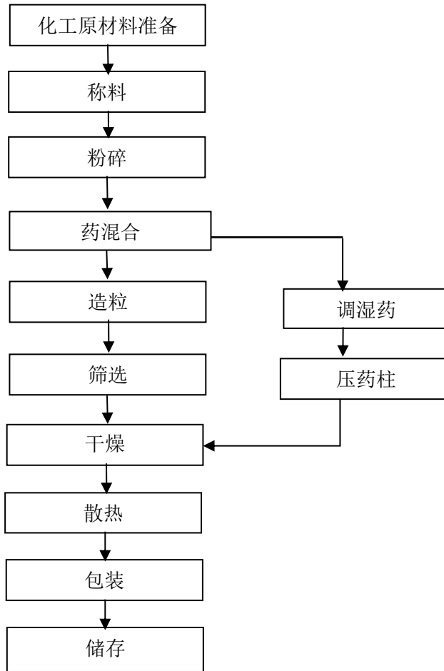
图 2.6-1 亮珠、药柱生产工艺流程图
