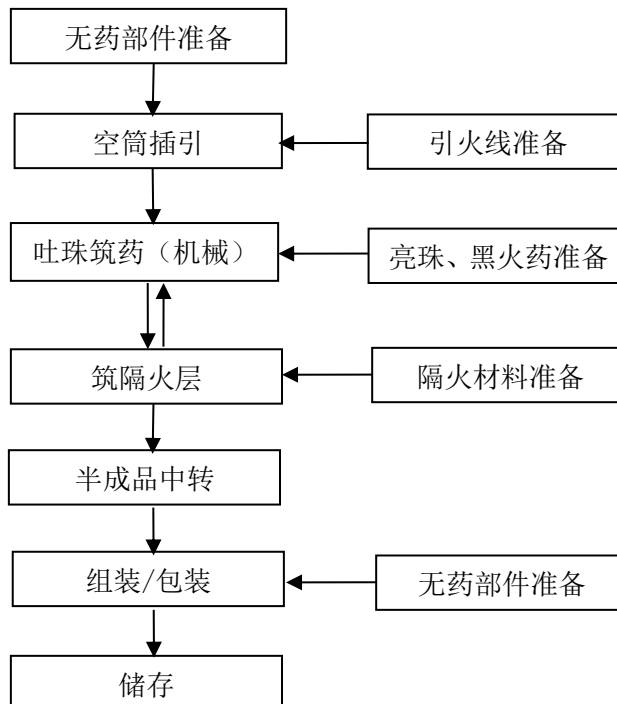
图 2.6-2 吐珠类产品生产工艺流程图
