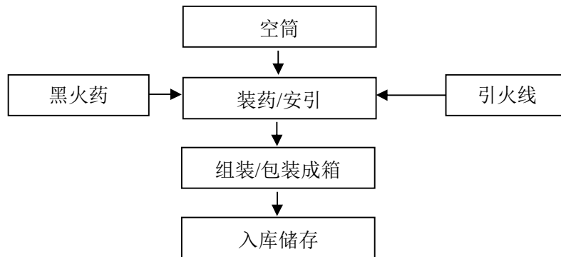
图 2.3-3：玩具类（玩具造型-地雷炮）生产工艺流程图
