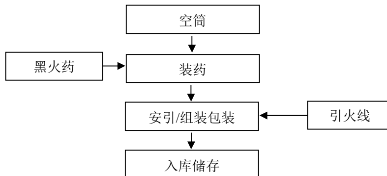
图 2.3-4：玩具类（玩具造型-青蛙炮）生产工艺流程图
