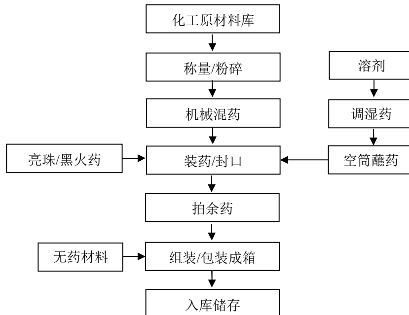
图 2.3-1：玩具类（线香型—晨光花）生产工艺流程图
