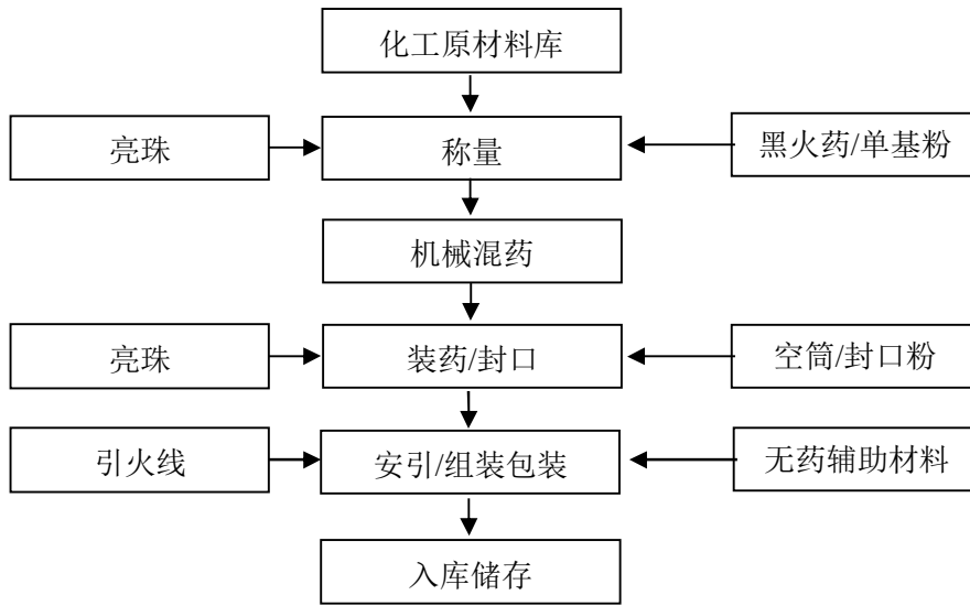
图 2.3-5：喷花类产品生产工艺流程图
