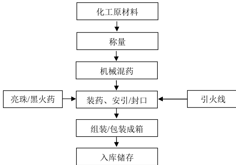
图 2.3-2：玩具类（玩具造型-坦克）等生产工艺流程图
