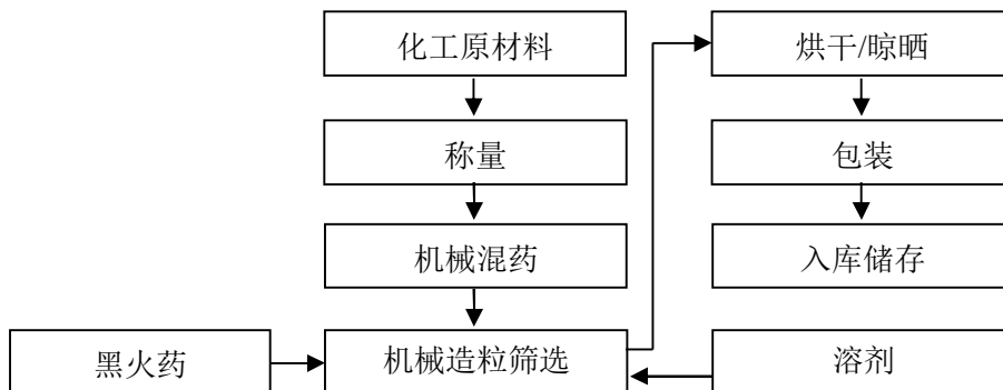
图 2.3-7：亮珠生产工艺流程图
