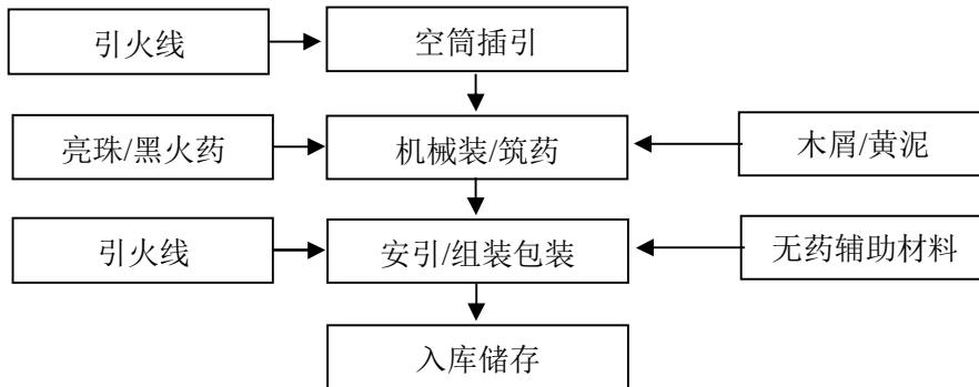
图 2.3-6：吐珠类产品生产工艺流程图
