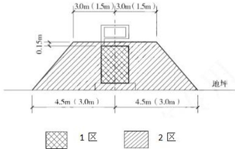
图3.10-2 汽油加油机爆炸危险区域划分
