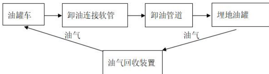
图 2.2-1 汽油加油工艺流程图
