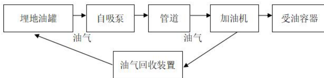
图 2.2-2 汽油卸油工艺流程图
